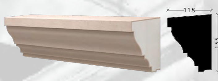
MP-97 - 155x118x1500 mm
