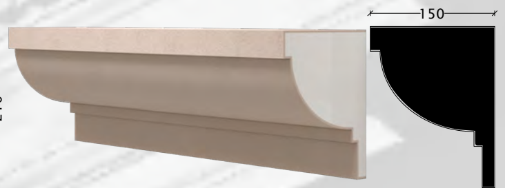
CG-58 - 195x150x1500 mm
