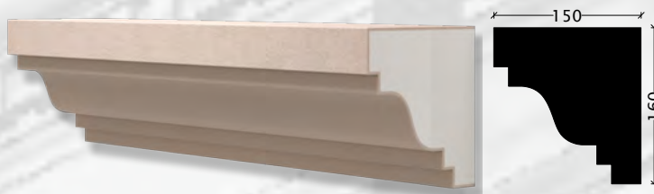
CG-35 - 160x150x1500 mm
